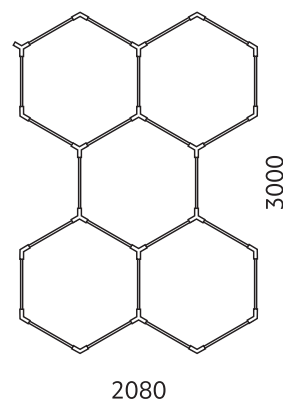
ŁĄCZNIK Y HEXLINE / CONNECTOR Y HEXLINE
