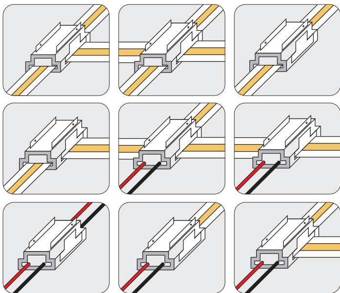
ŁĄCZNIK/CONNECTOR „9w1”
