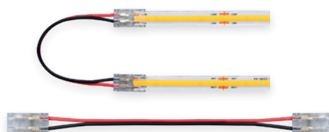
ŁĄCZNIK DWUSTRONNY 10 cm / DOUBLE-SIDED CONNECTOR 10 cm
