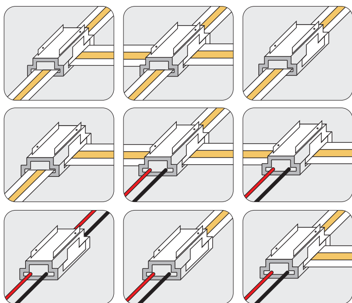
ŁĄCZNIK/CONNECTOR „9w1”
